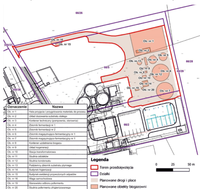
Planowane zagospodarowanie terenu - obiekty biogazowni na oczyszczalni w Bytkowie
