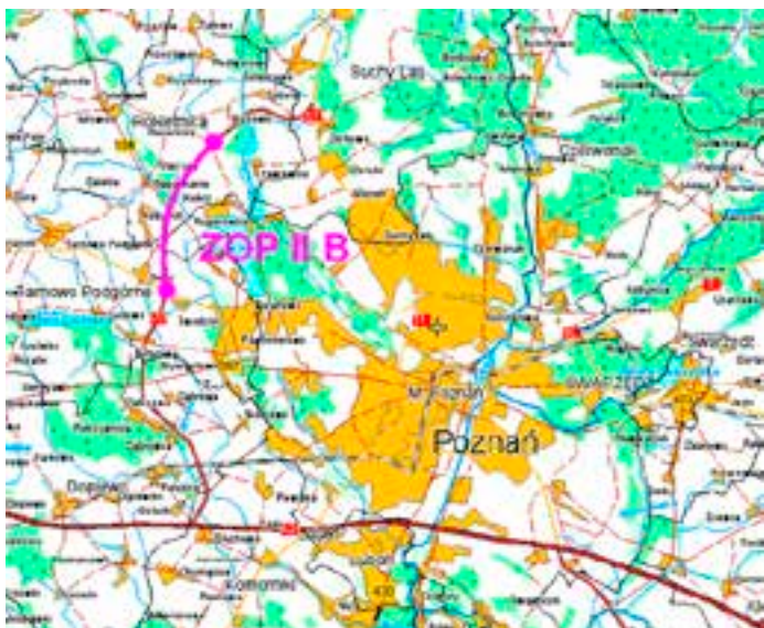
Węzeł Kobylniki (styk z drogą wojewódzka 184) z dwoma rondami : http://www.s11rokietnica-swadzim.pl/opis.html
