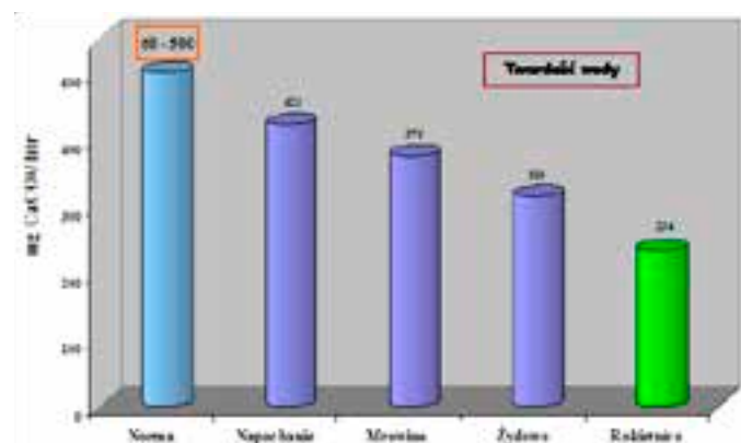
Ryc. 8. Porównanie zawartości „Żelaza” w wodzie gminnej z normą (Rozporządzenia Ministra Zdrowia z dnia 29 marca 2007 r.)
