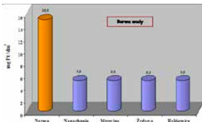
Ryc. 5. Porównanie „Barwy” wody gminnej z normą (Rozporządzenia Ministra Zdrowia z dnia 29 marca 2007 r.)
