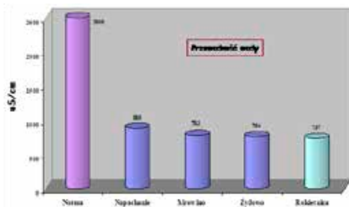
Ryc. 6. Porównanie „Przewodności” wody gminnej z normą (Rozporządzenia Ministra Zdrowia z dnia 29 marca 2007 r.)
